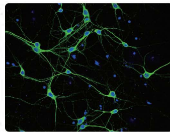
MAP2 antibody (GTX133109)
